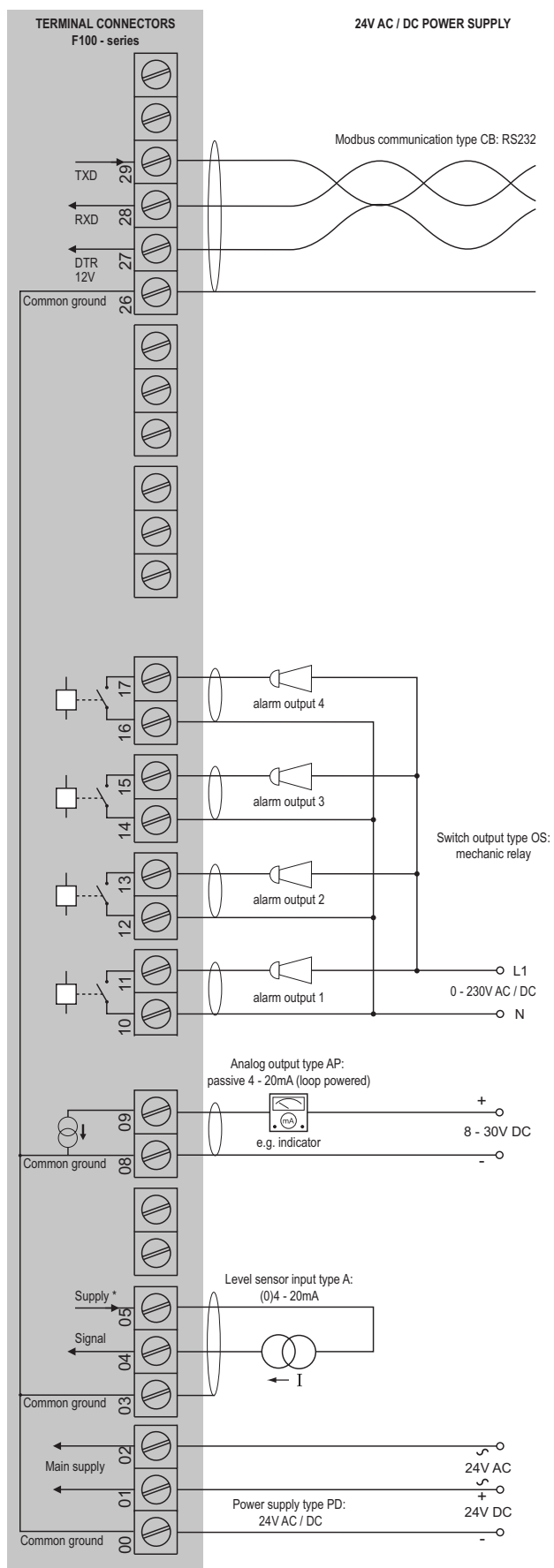
Configuration example F170-A-AP-CB-OS-PD-XX-ZX
